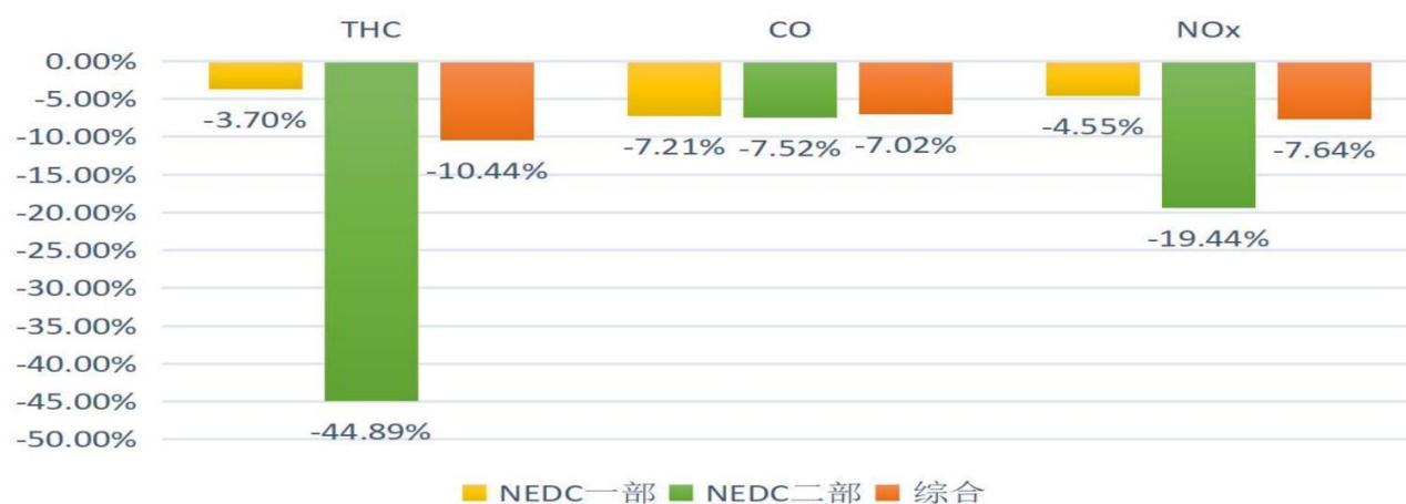
汽油车试验结果
